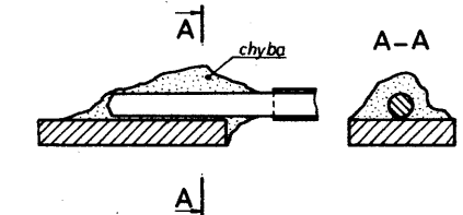
Obr. 6. Mezní případ k obr. 5 — pájený spoj s maximálně přípustným množstvím pájky. Konec uloženého vodiče musí být zřetelně rozpoznatelný. Mezní případy „Pájený spoj s minimálně přípustným množstvím pájky“ a „Pájený spoj s omezenou chybou smáčení“ nejsou u pájení podle obr. 5 přípustné, vzhledem k nedostatečné mechanické pevnosti výsledného spoje při těchto chybách
